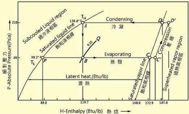
冷媒莫里爾(P-H)圖
